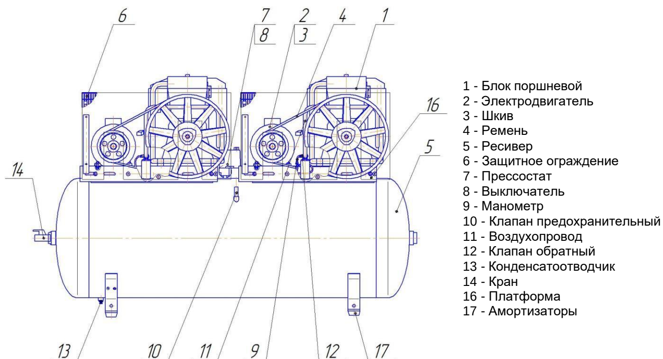
Рисунок 11 - Общий вид компрессора СБ4/Φ-500.AB858TB
