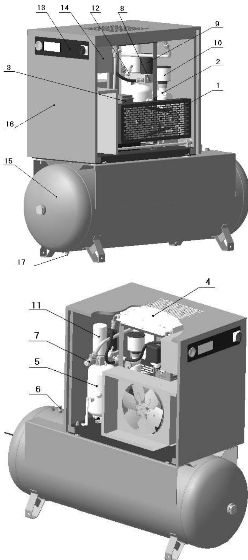
Рисунок 2 – Общий вид компрессорной установки BK15T-...-500
